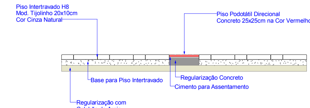
Det. Passeio/Piso Tátil ESC.: 1: 20
