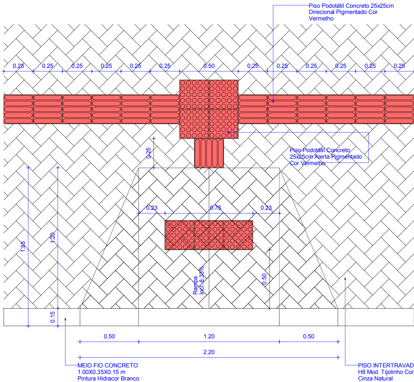
Det. Rampa Acessibilidade ESC.: 1: 20
