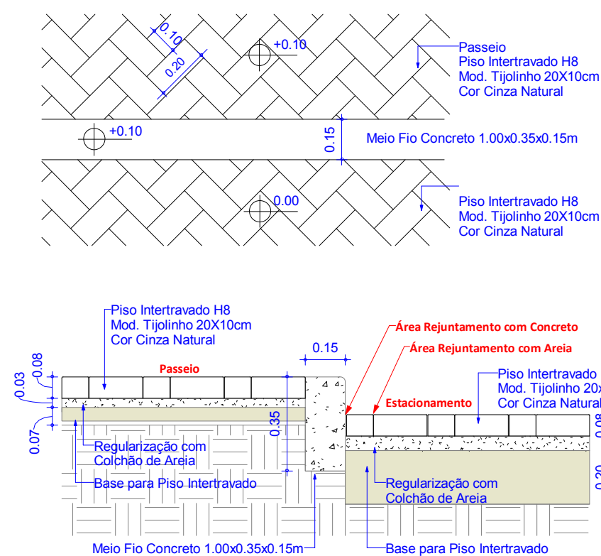
Det. Meio Fio ESC.: 1: 20
