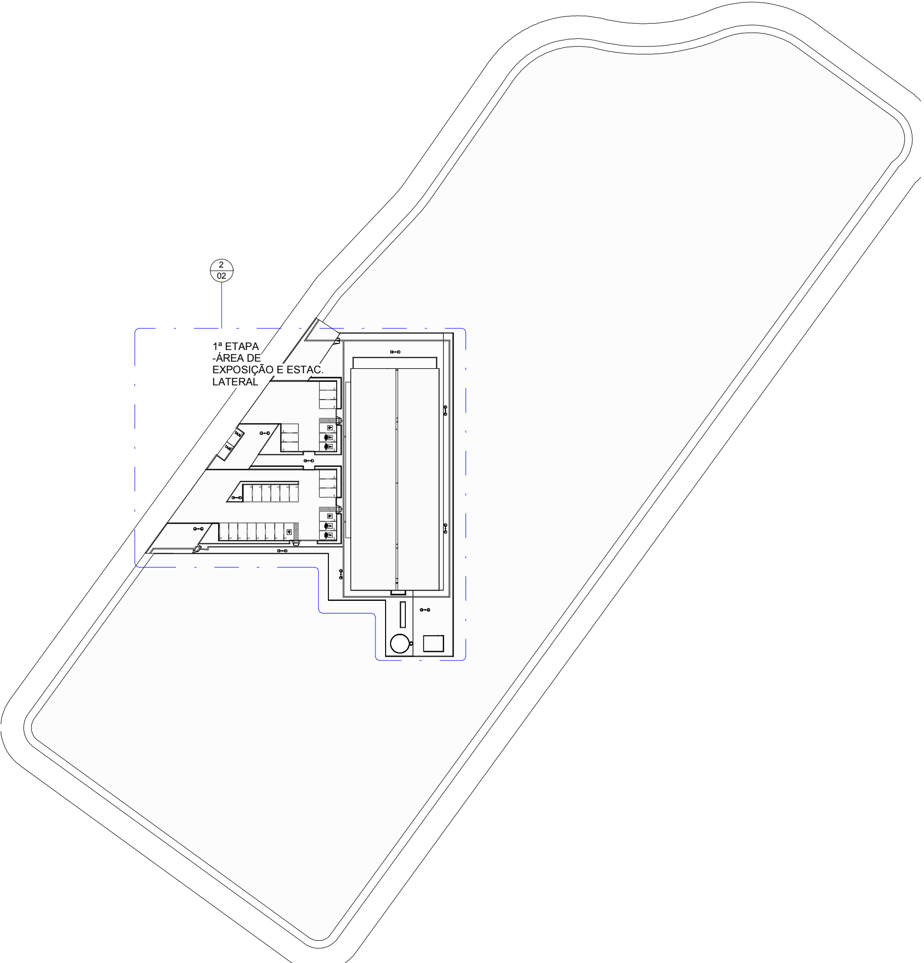
1 PI Urbanização/Área Permeável/Estacionamento-Setores ESC.: 1: 1000
