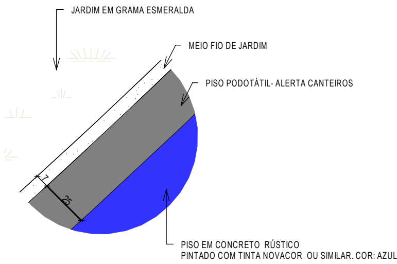
2 DETALHE MEIO FIO DE JARDIM 1: 20
