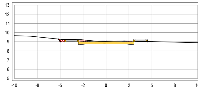
SEÇÃO TRANSVERSAL: 10+0
