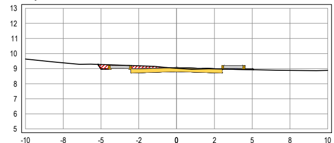
SEÇÃO TRANSVERSAL: 10+10
