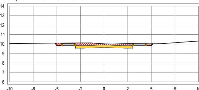
SEÇÃO TRANSVERSAL: 13+10
