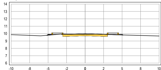
SEÇÃO TRANSVERSAL: 9+0
