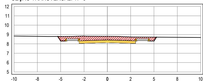
SEÇÃO TRANSVERSAL: 17+0
