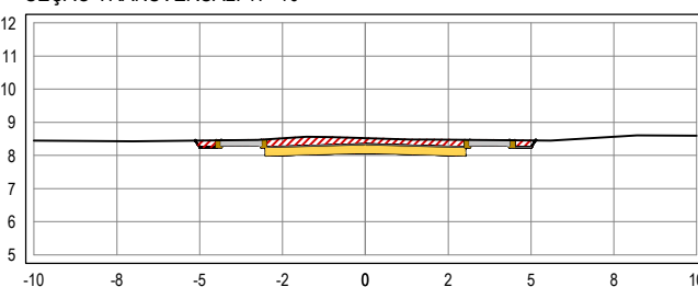
SEÇÃO TRANSVERSAL: 17+10
