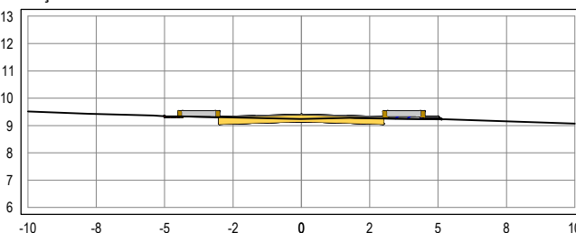
SEÇÃO TRANSVERSAL: 9+10
