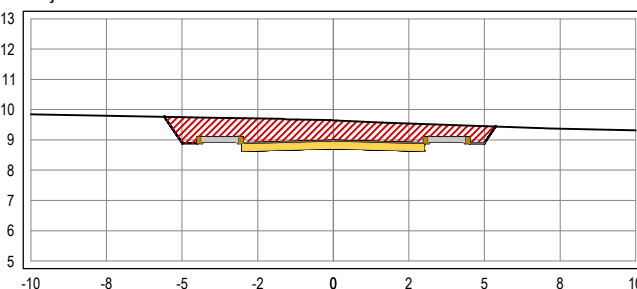
SEÇÃO TRANSVERSAL: 15+10
