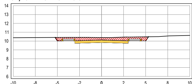
SEÇÃO TRANSVERSAL: 13+0
