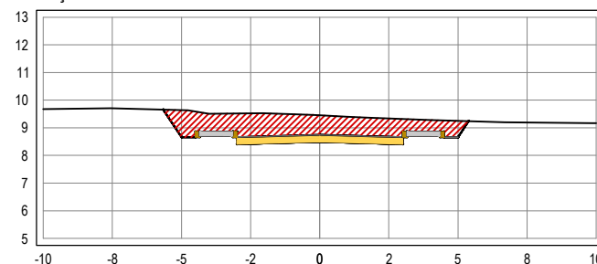
SEÇÃO TRANSVERSAL: 16+0
