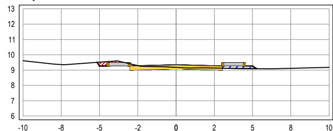
SEÇÃO TRANSVERSAL: 11+0
