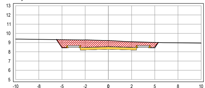
SEÇÃO TRANSVERSAL: 16+10
