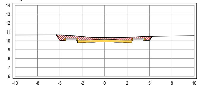
SEÇÃO TRANSVERSAL: 12+10
