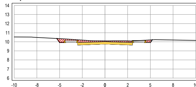
SEÇÃO TRANSVERSAL: 12+0
