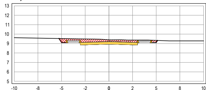
SEÇÃO TRANSVERSAL: 15+0
