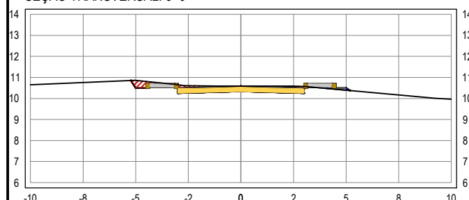
SEÇÃO TRANSVERSAL: 6+0
