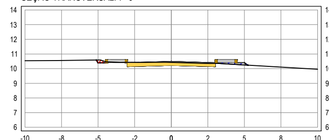
SEÇÃO TRANSVERSAL: 7+0
