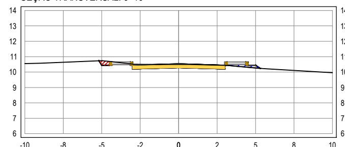
SEÇÃO TRANSVERSAL: 6+10
