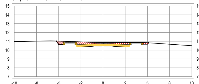
SEÇÃO TRANSVERSAL: 4+10
