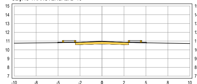
SEÇÃO TRANSVERSAL: 2+10
