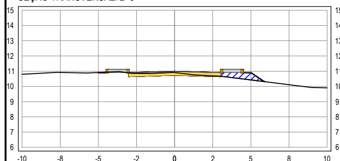
SEÇÃO TRANSVERSAL: 2+0
