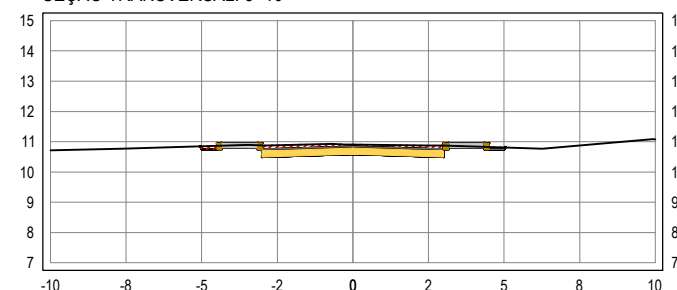
SEÇÃO TRANSVERSAL: 3+10
