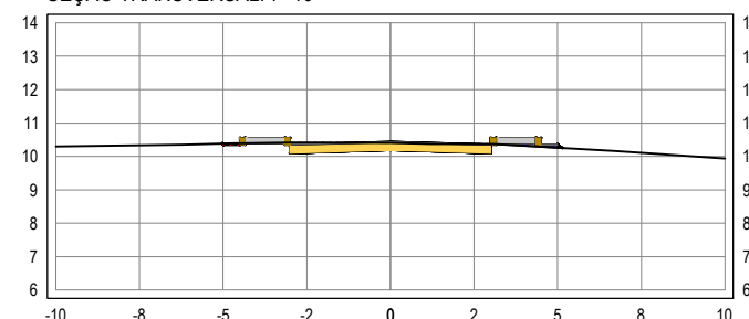
SEÇÃO TRANSVERSAL: 7+10
