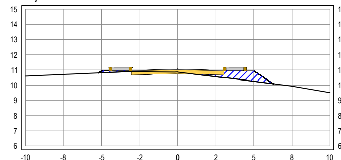
SEÇÃO TRANSVERSAL: 1+10
