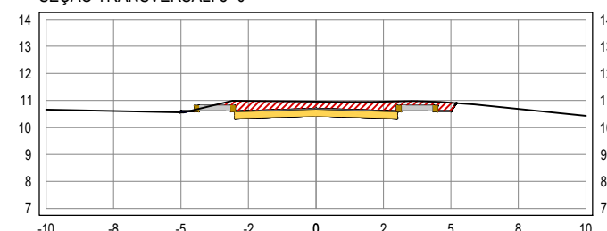
SEÇÃO TRANSVERSAL: 5+0
