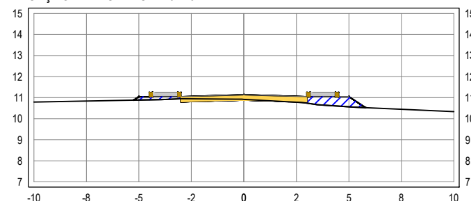
SEÇÃO TRANSVERSAL: 0+10
