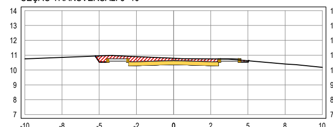
SEÇÃO TRANSVERSAL: 5+10
