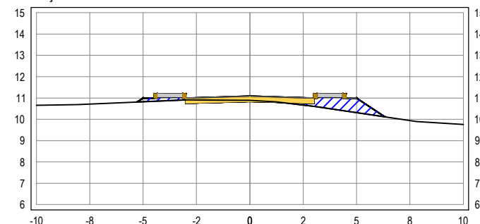
SEÇÃO TRANSVERSAL: 1+0
