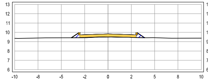
SEÇÃO TRANSVERSAL: 2+0
