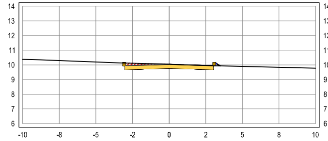
SEÇÃO TRANSVERSAL: 0+0
