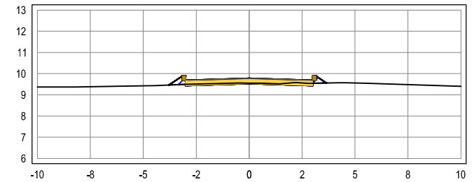
SEÇÃO TRANSVERSAL: 2+10
