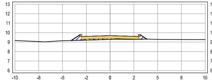
SEÇÃO TRANSVERSAL: 4+11
