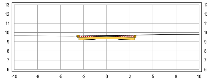
SEÇÃO TRANSVERSAL: 4+10
