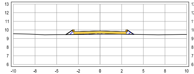
SEÇÃO TRANSVERSAL: 1+10
