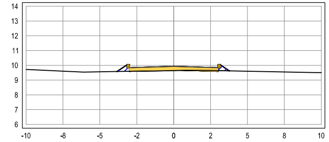
SEÇÃO TRANSVERSAL: 1+0
