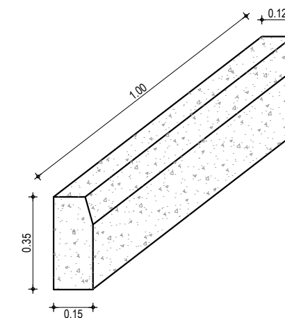
02 DETALHE MEIO FIO SEM ESCALA
