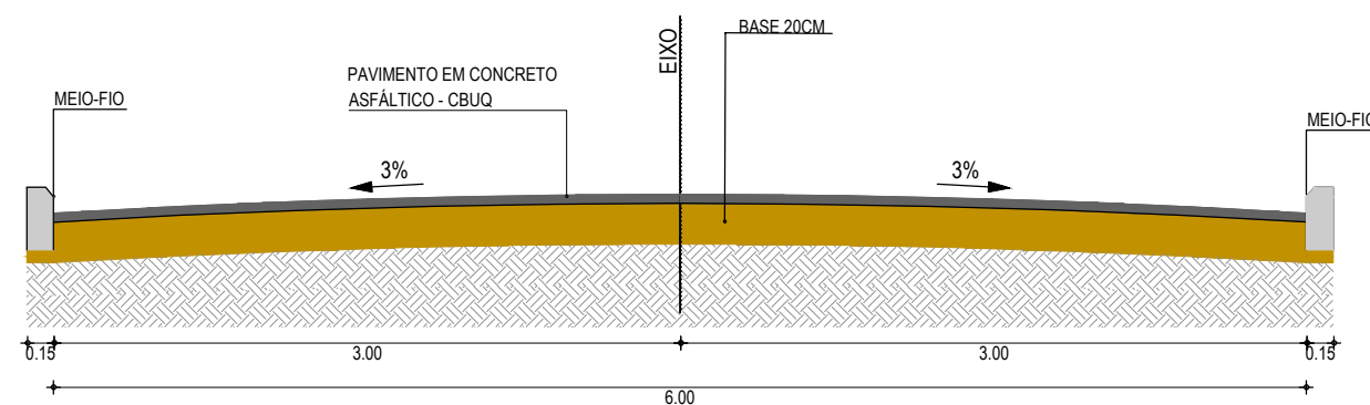
01 SEÇÕES TIPO SEM ESCALA
