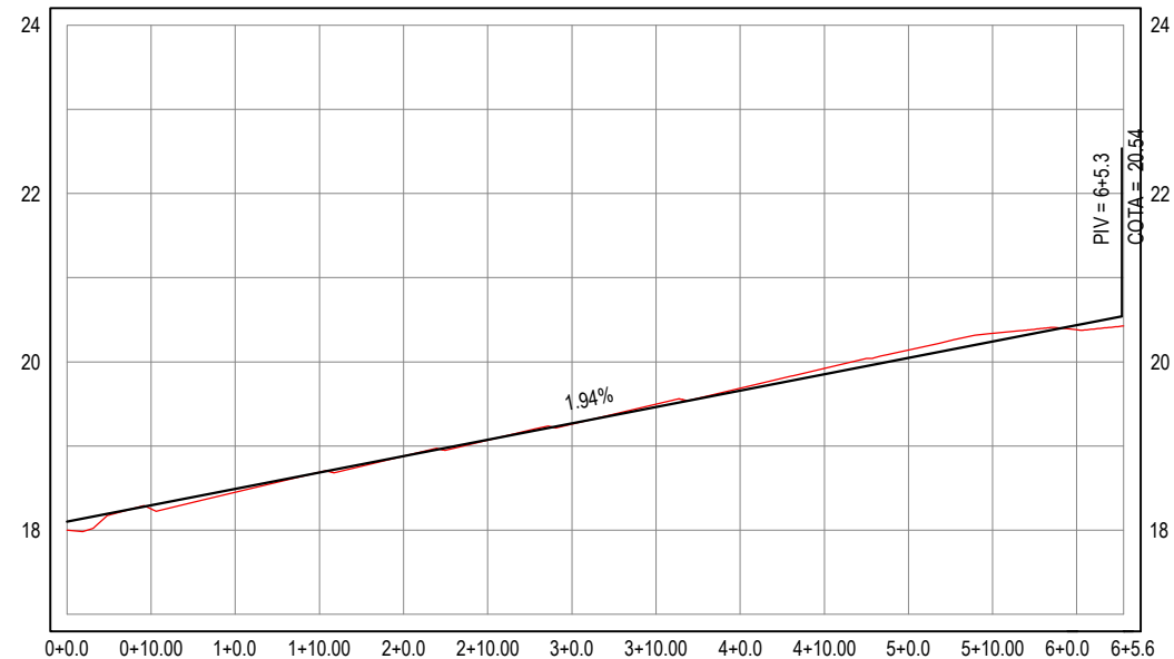
PERFIL: RUA VALDEMAR ELISARIO
