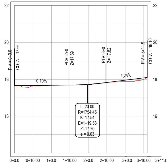
PERFIL: RUA NOGUEIRA DA COSTA
