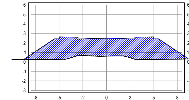
SEÇÃO TRANSVERSAL: 13+0
