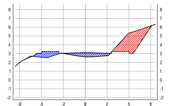
SEÇÃO TRANSVERSAL: 11+0
