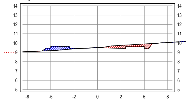
SEÇÃO TRANSVERSAL: 0+0
