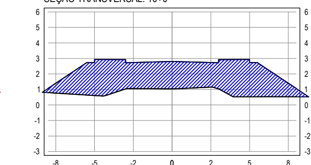
SEÇÃO TRANSVERSAL: 10+0
