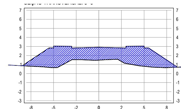
SEÇÃO TRANSVERSAL: 13+0
