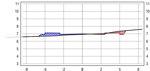
SEÇÃO TRANSVERSAL: 3+0
