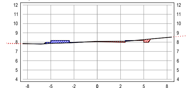
SEÇÃO TRANSVERSAL: 2+0
