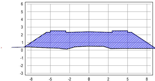
SEÇÃO TRANSVERSAL: 14+0
