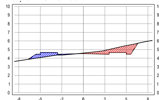
SEÇÃO TRANSVERSAL: 8+0
