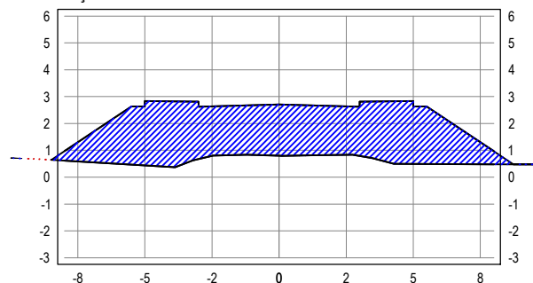
SEÇÃO TRANSVERSAL: 11+0
