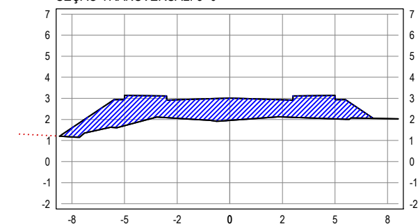
SEÇÃO TRANSVERSAL: 8+0
